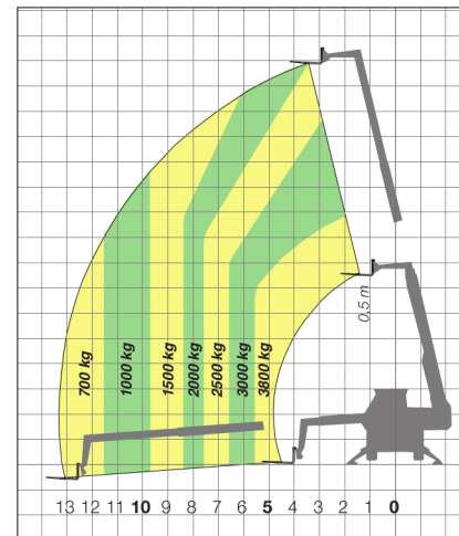
ROTO 38.16 / ROTO 38.16 S FORCHE SU STABILIZZATORI SU 360°
