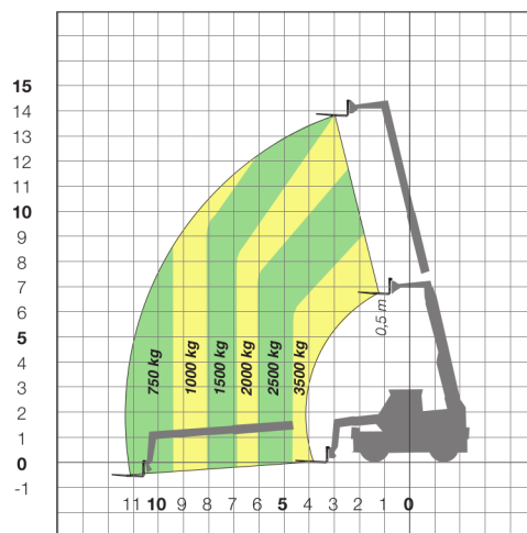
ROTO 38.14 / ROTO 38.14 S FORCHE SU PNEUMATICI FRONTALE
