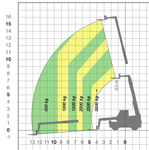
ROTO 38.16 / ROTO 38.16 S FORCHE SU PNEUMATICI FRONTALE
