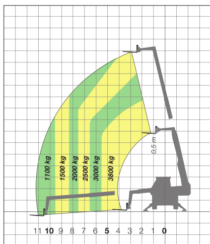
ROTO 38.14 / ROTO 38.14 S FORCHE SU STABILIZZATORI SU 360°
